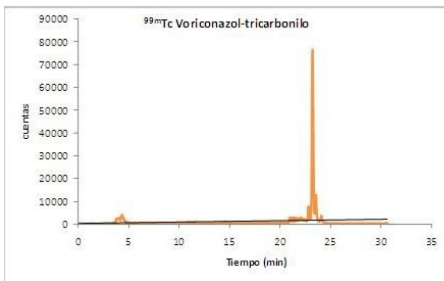
Figura 4.- Cromatograma del 99mTc voriconazol-tricarbonilo.
