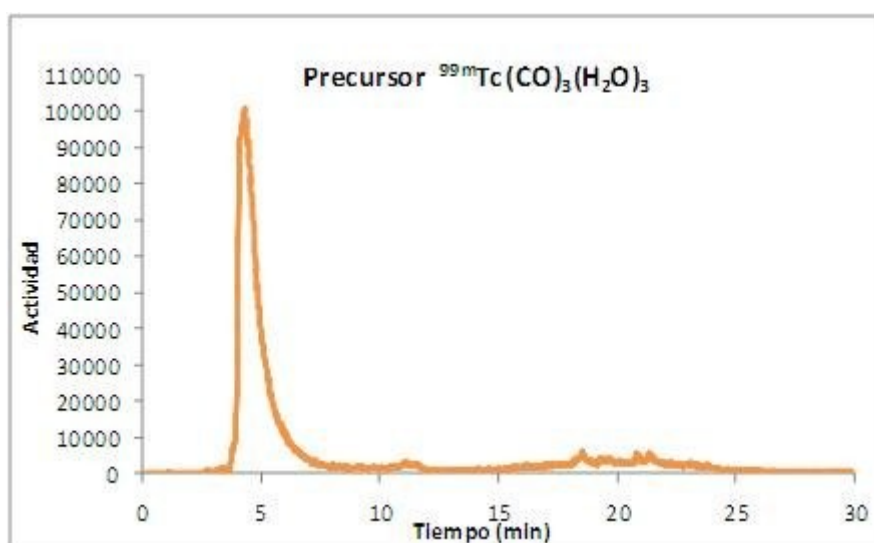
Figura 3.- Cromatograma del precursor tricarbonílico.
