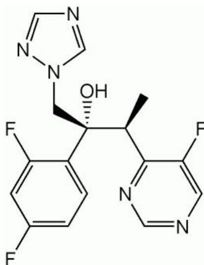
Figura 1.- Voriconazol: 2-(2,4-Difluoro-fenil)-3-(fluoropirimidin-4-yl)-1-[1, 2,4] triazol-1-yl-butan-2-ol.
